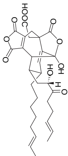
phomoidride A (1)
